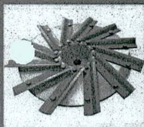
Rotor com 12 facas picadoras e 6 lançadores. (Sistema quebra grãos)
