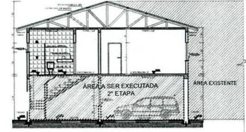
CORTE AA'
