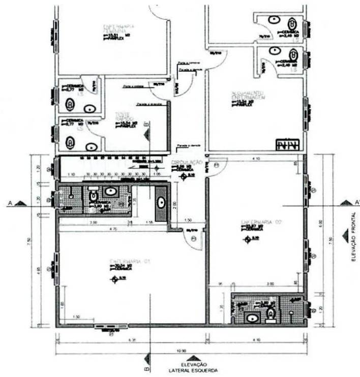
PLANTA BAIXA - PAVIMENTO TÉRREO
