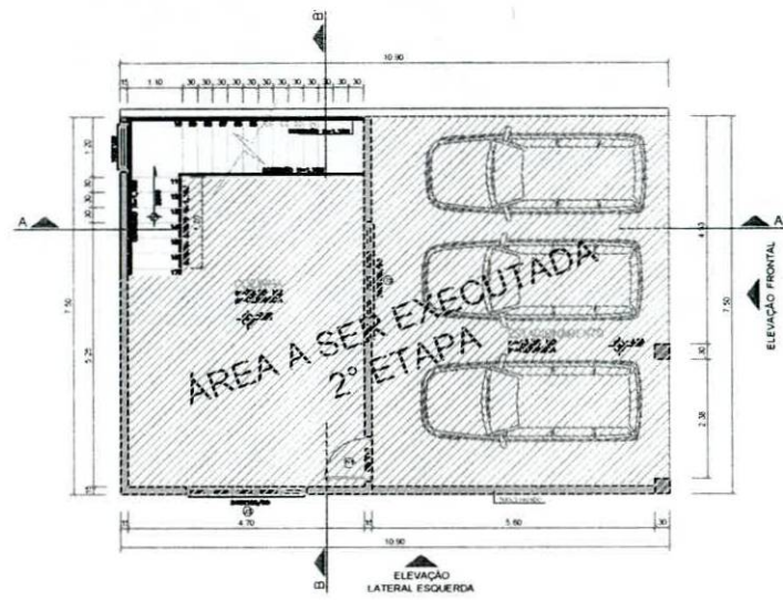
PLANTA BAIXA - SUBSOLO
