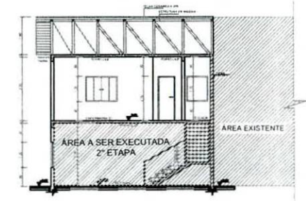
CORTE BB'
