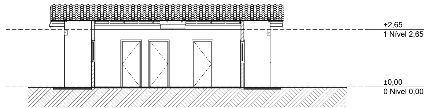
Corte 1:100
