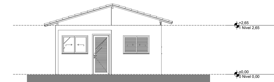
Elevação Frontal 1:100
