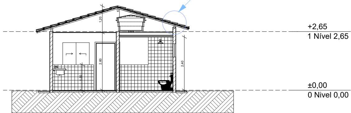
Corte 1:100
