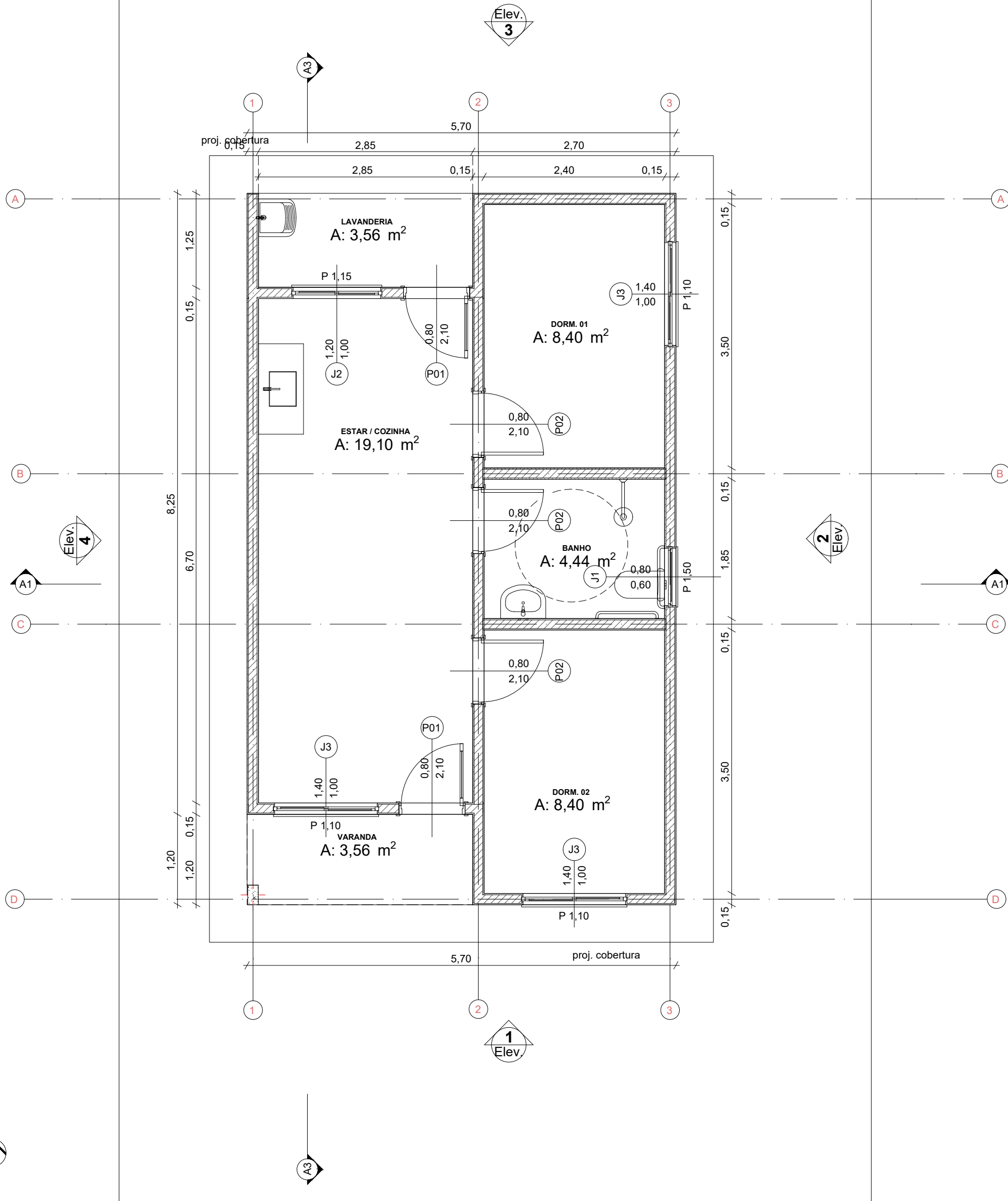
Planta Térreo 1:50
