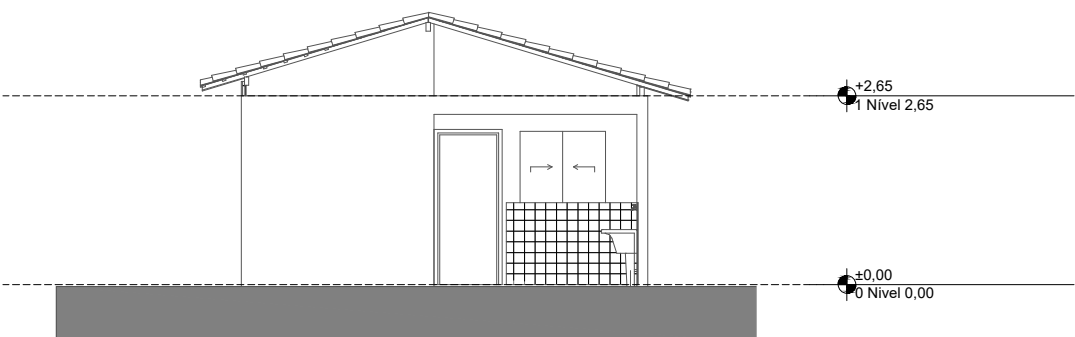
Elevação Posterior 1:100
